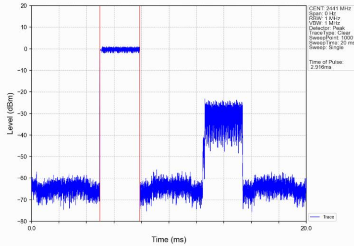
8DPSK_3DH5_HOPP_Ant1_NTNV
