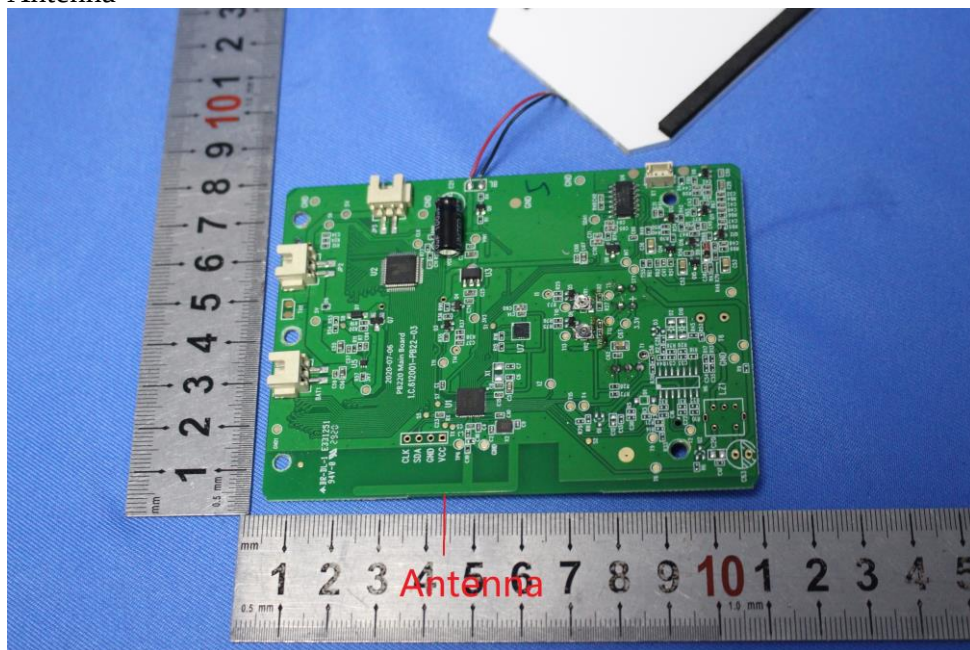
Antenna
