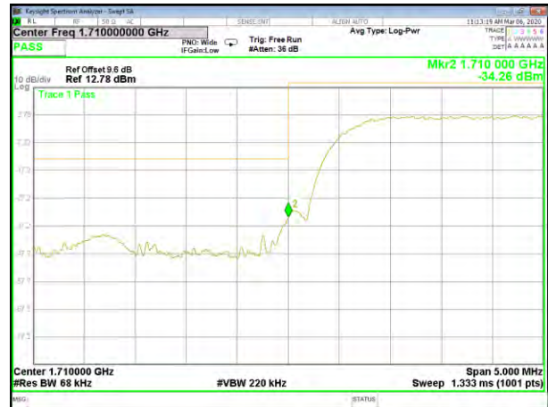
B4_HSDPA_Lower_Band edge
