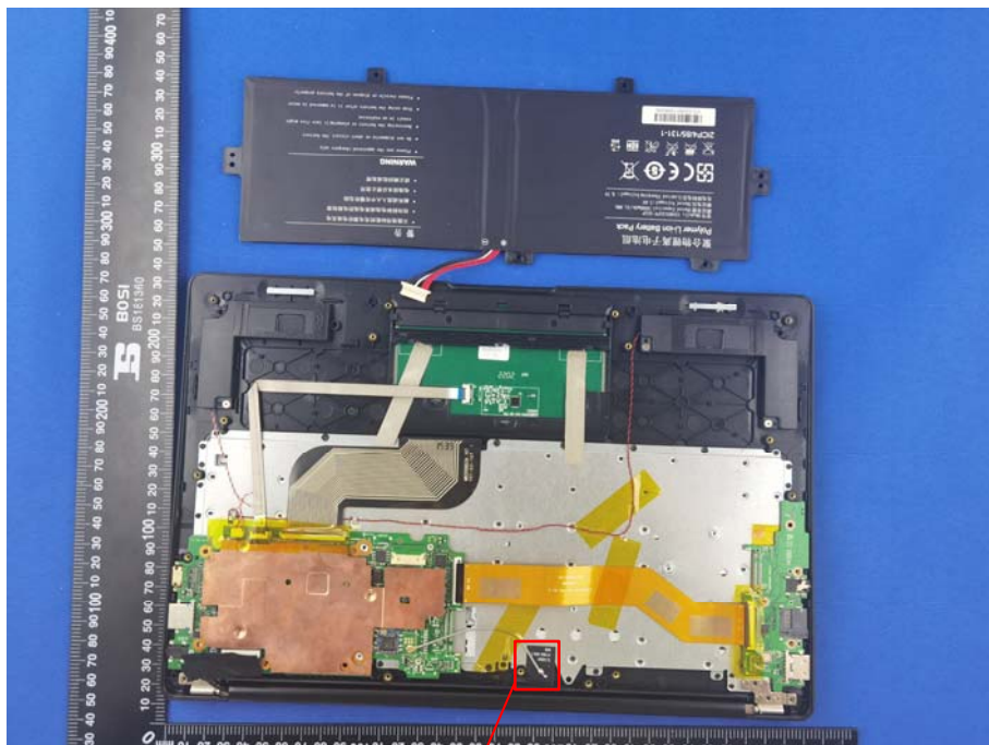
PIFA Antenna
