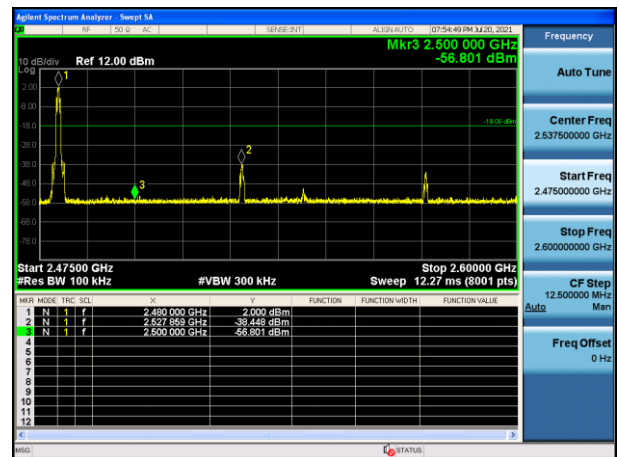
Mode 2 CH78(2480MHz)
