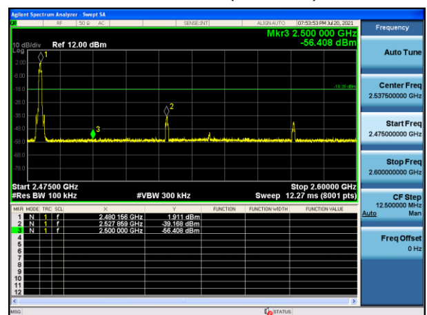
Mode 3 CH78(2480MHz)
