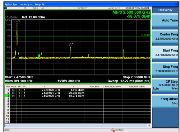
Mode 1 CH78(2480MHz)
