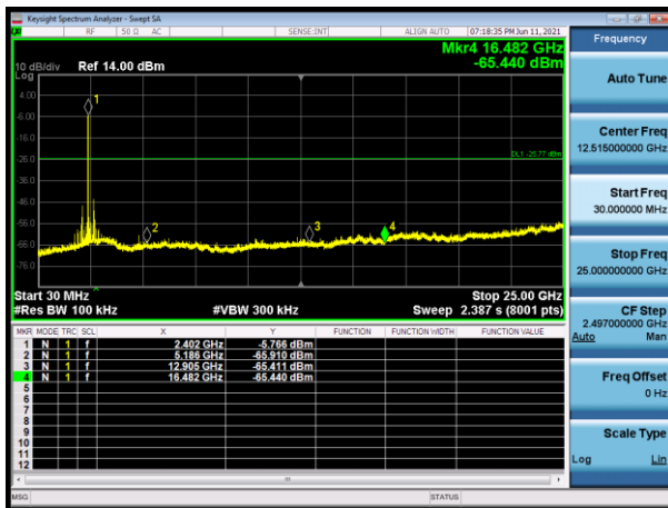
Mode 2 CH00(2402MHz)
