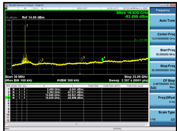
Mode 3 CH78(2480MHz)
