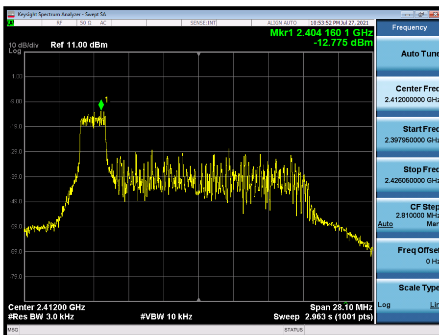
Mode 4 2412MHz
