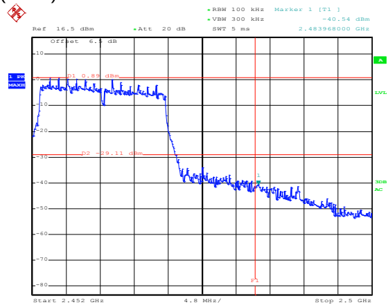
802.11n(HT20)
