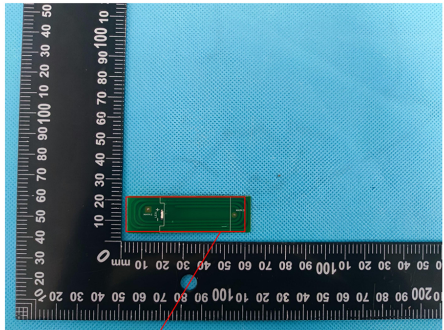
NFC Antenna
