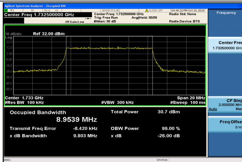
Band4-10MHz-QPSK-20175-50RB#0-8.9539
