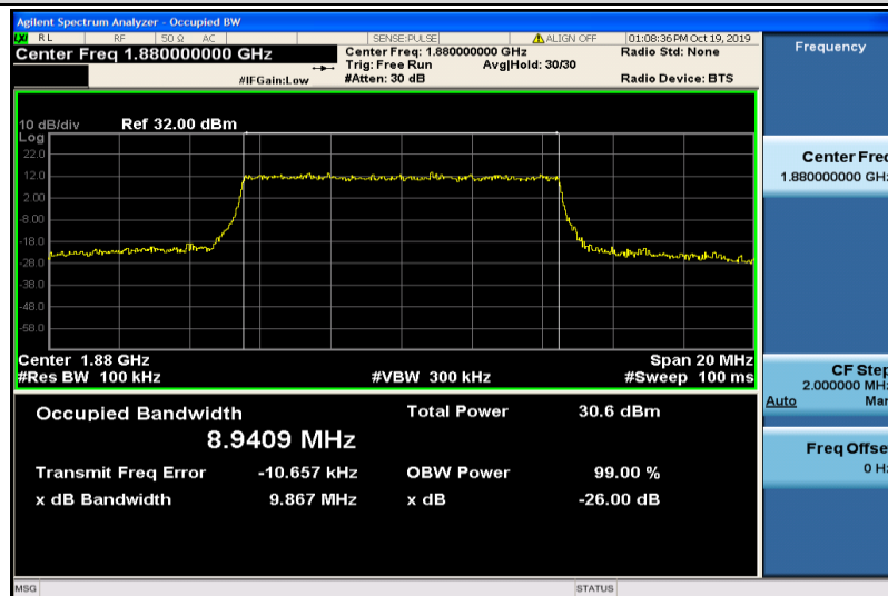
Band2-10MHz-QPSK-18900-50RB#0-8.9409
