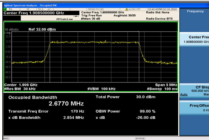
Band2-3MHz-QPSK-19185-15RB#0-2.6770
