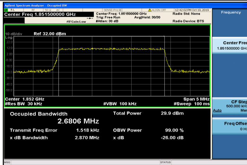
Band2-3MHz-QPSK-18615-15RB#0-2.6806
