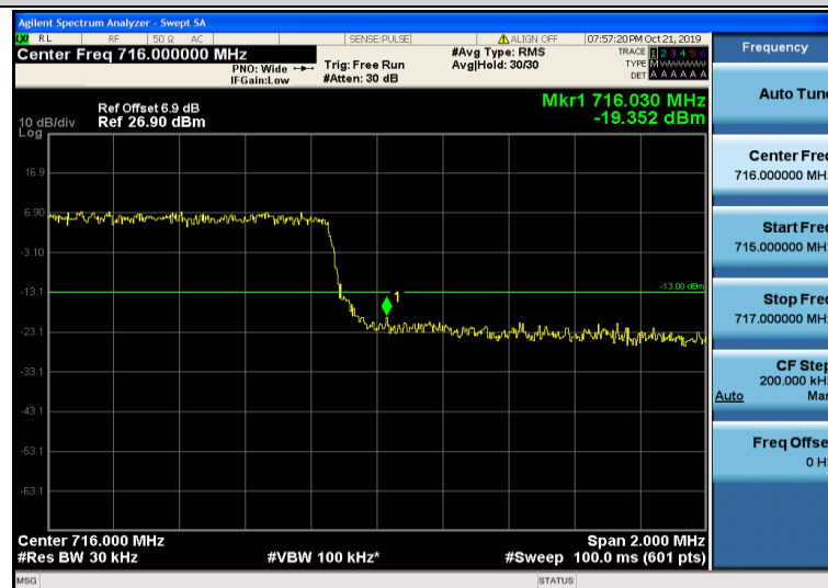
Band12-3MHz-QPSK-23165-15RB#0
