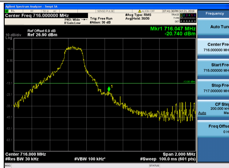
Band12-3MHz-QPSK-23165-1RB#14
