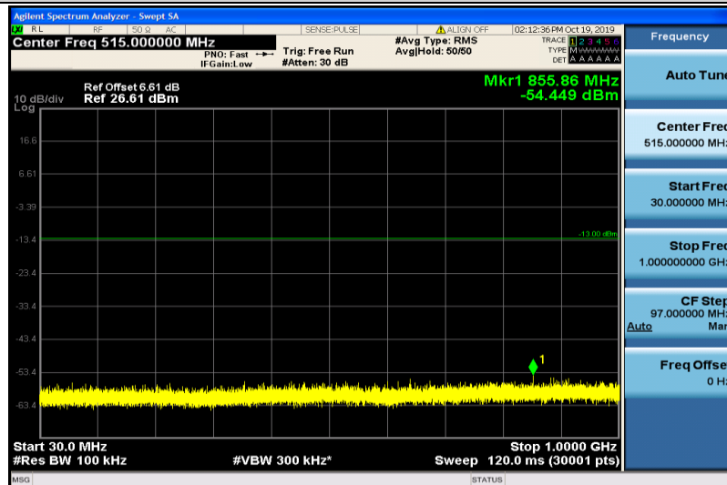
Band2-3MHz-QPSK-18900-1RB#0-30~1000MHz
