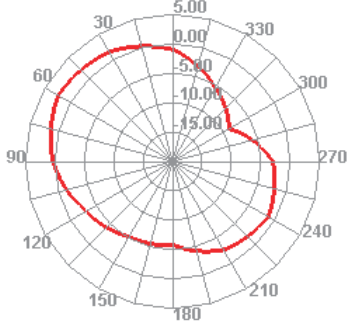
2450.000MHz H
