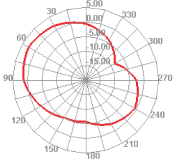
2500.000MHz H
