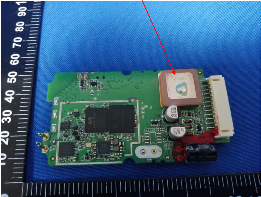
GPS ANT
