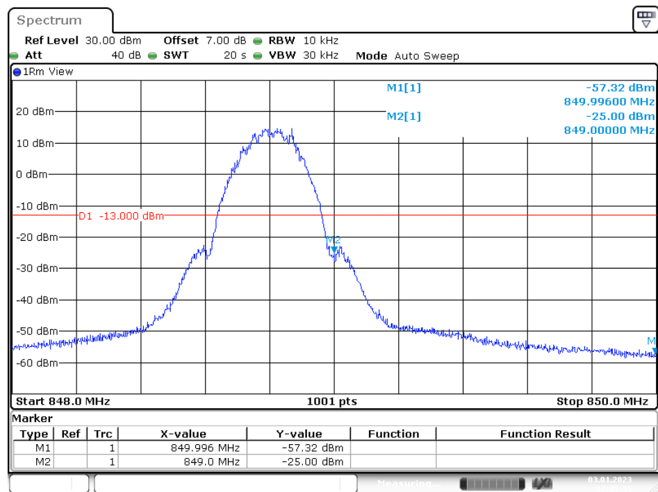
Right Band Edge for GSM (GMSK) Mode
