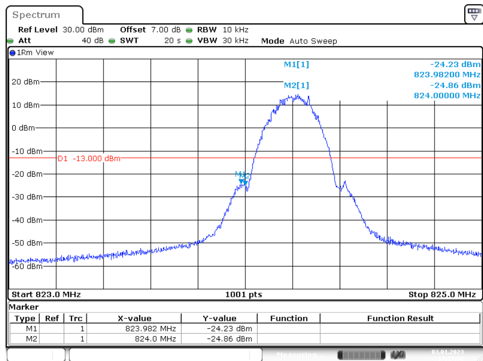
Left Band Edge for GSM (GMSK) Mode
