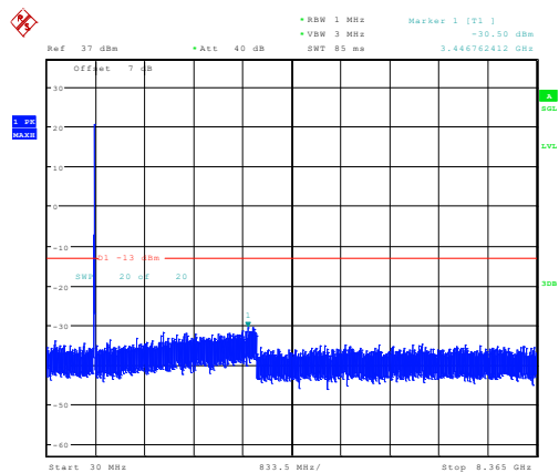
10MHz_Middle_QPSK_50@0 -30.50dBm
