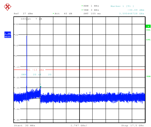
10MHz_High_QPSK_50@0 -30.09dBm
