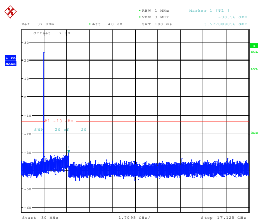
5MHz_Low_QPSK_25@0 -30.56dBm
