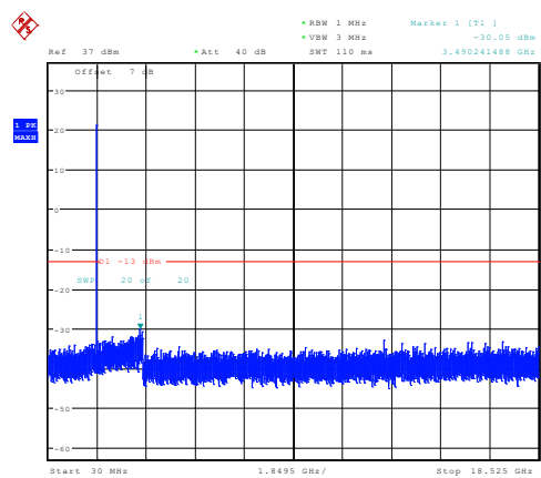
5MHz_Low_QPSK_1@0 -30.05dBm
