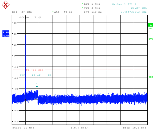
10MHz_Middle_QPSK_50@0 -29.27dBm
