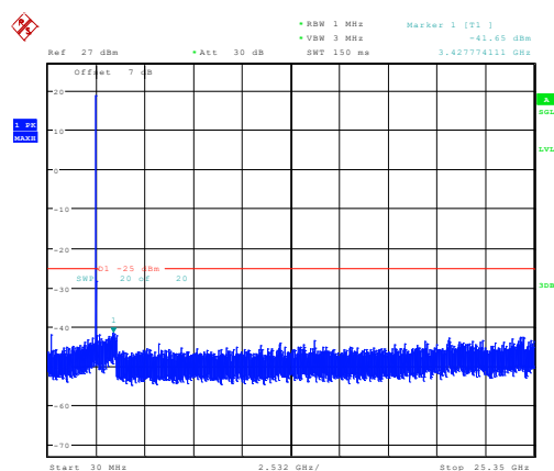
10MHz_Middle_QPSK_1@0 -41.65dBm
