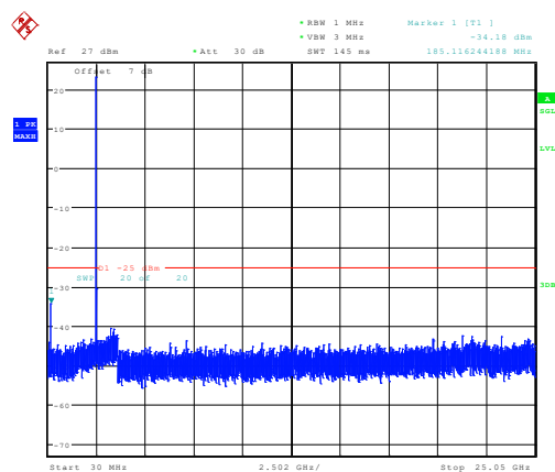
10MHz_Low_QPSK_1@0 -34.18dBm
