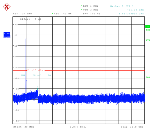
20MHz_Middle_QPSK_1@0 -31.39dBm
