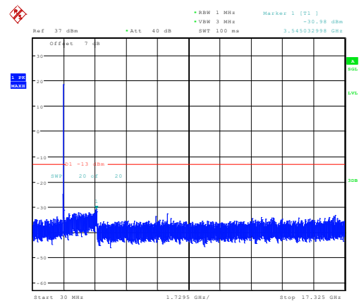
10MHz_Middle_QPSK_50@0 -30.98dBm
