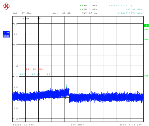
10MHz_Low_QPSK_50@0 -31.08dBm
