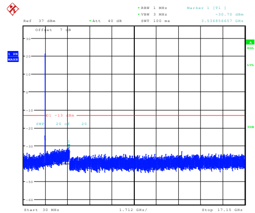
10MHz_Low_QPSK_50@0 -30.70dBm
