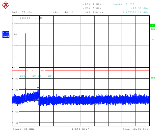
10MHz_Low_QPSK_50@0 -29.59dBm
