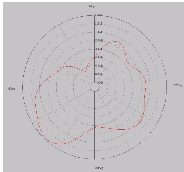
E2 plane
