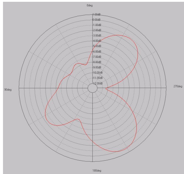
E2 plane
