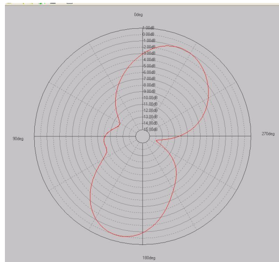
E2 plane
