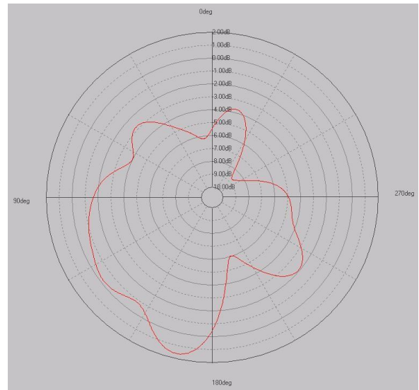
E2 plane
