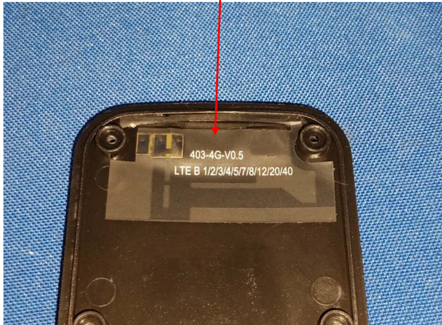
2G/4G ANT
