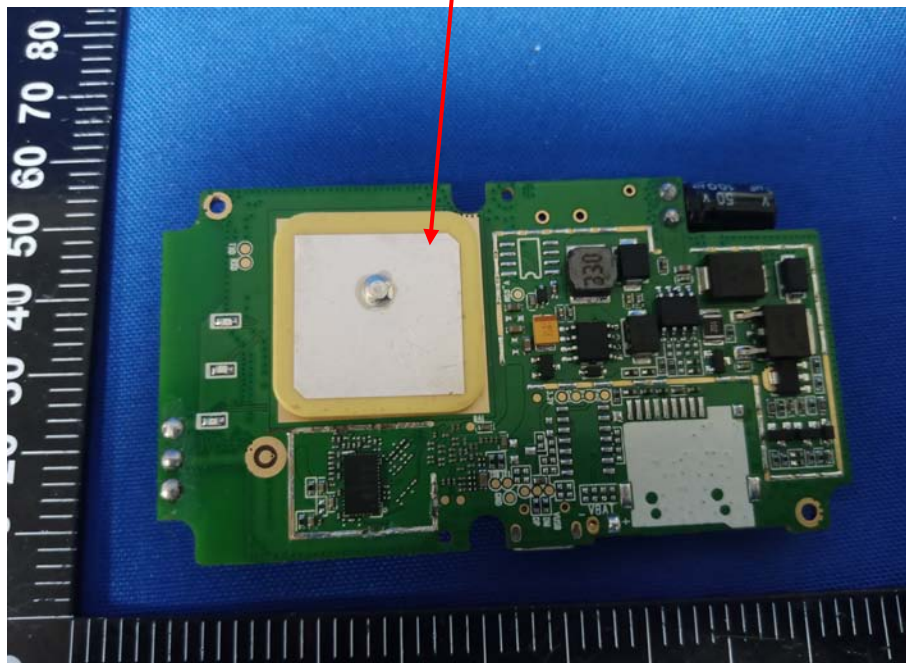
GPS ANT
