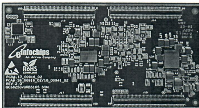
Bottom Side
