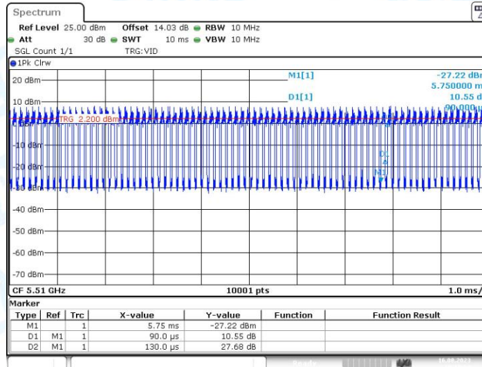
11AC40MIMO_Ant2_5510
