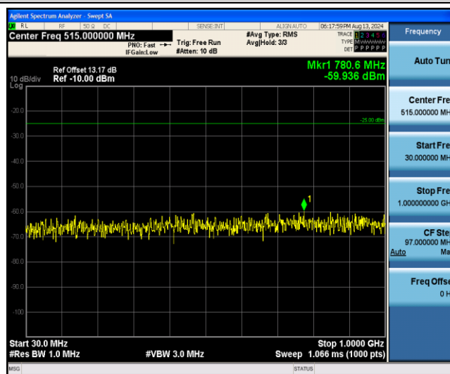
Band38-20MHz-QPSK-38150-1RB#0-Range4:1000~3000MHz
