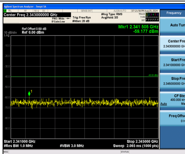
Band40-5MHz-QPSK-39200-1RB#0-Range5:2360~2365MHz
