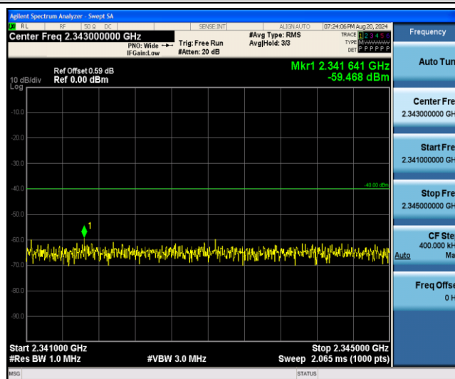
Band40-5MHz-QPSK-39225-1RB#0-Range5:2360~2365MHz
