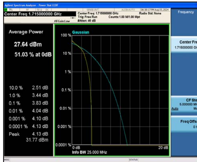
Band66-10MHz-QPSK-132022-50RB#0
