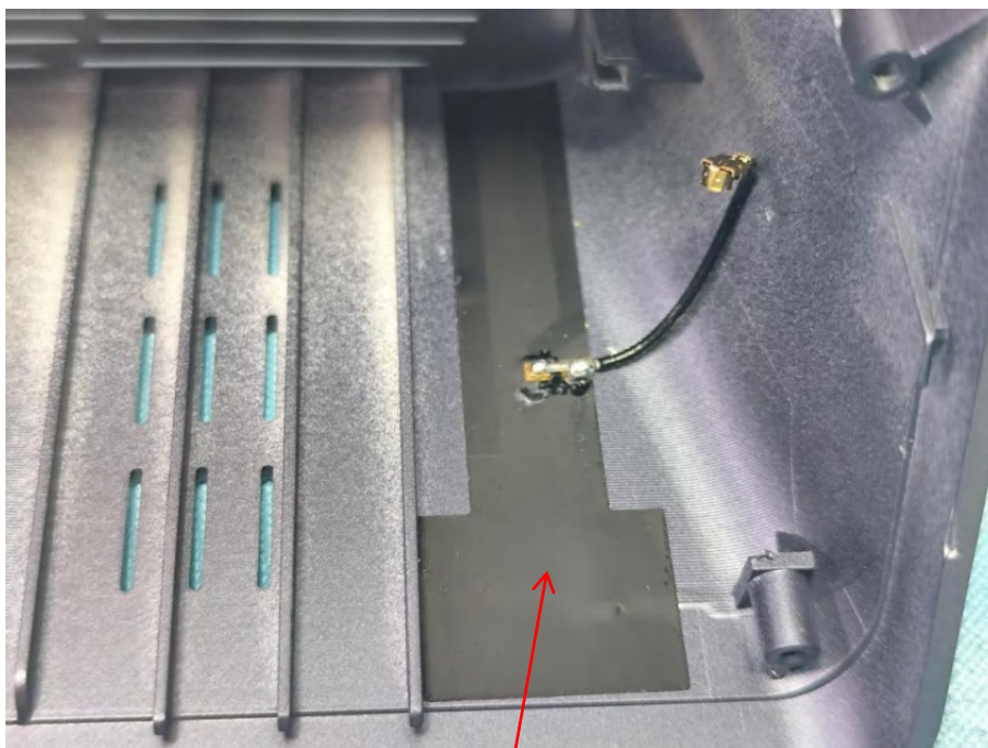
SRD ANT
