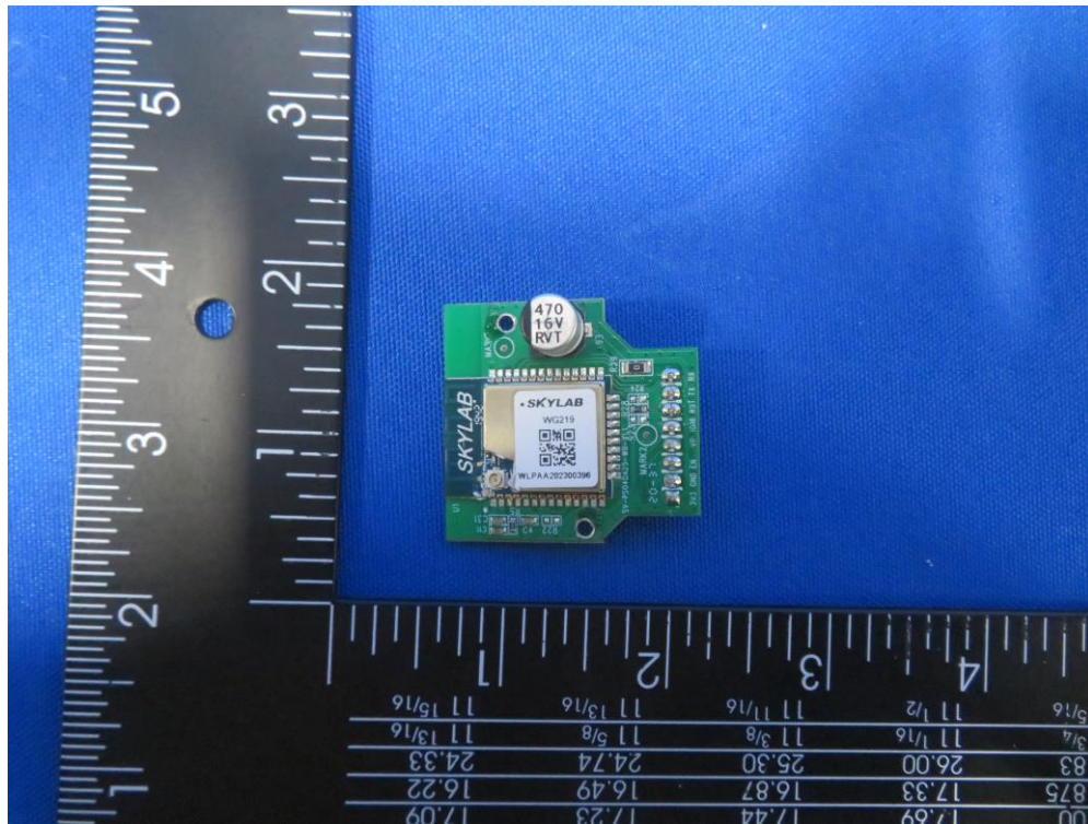
(9) EUT Photo
