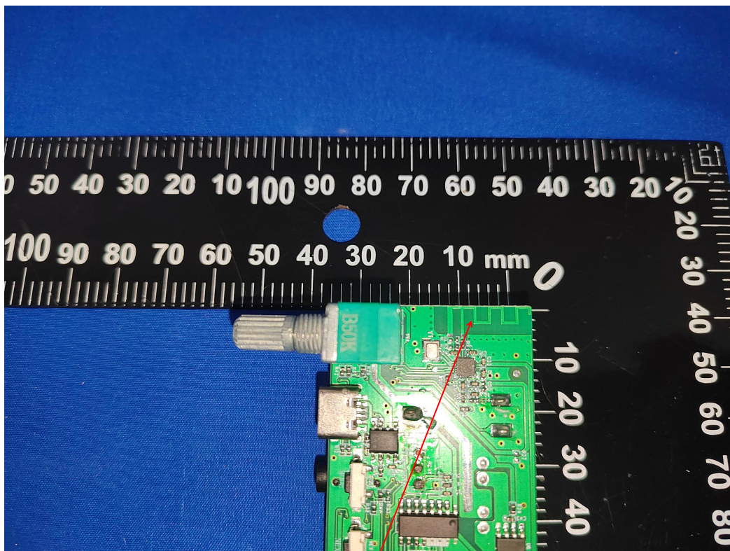
BT ANT 1
