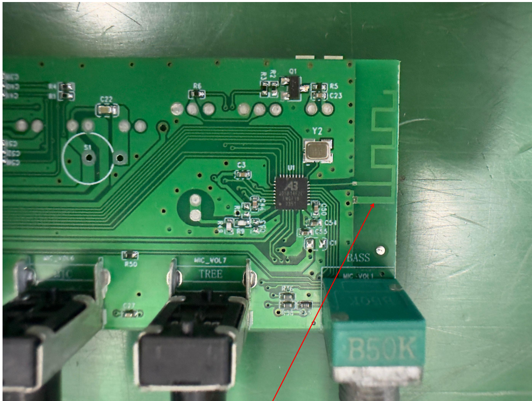
BT ANT 2
