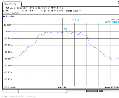
CH40
