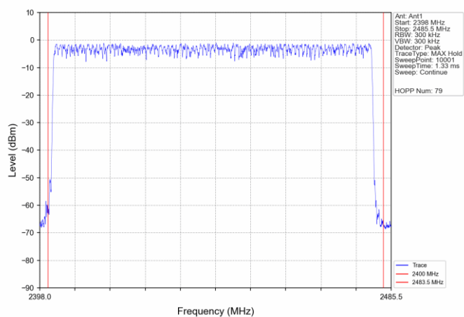
8DPSK_3DH5_HOPP_Ant1_NTNV
