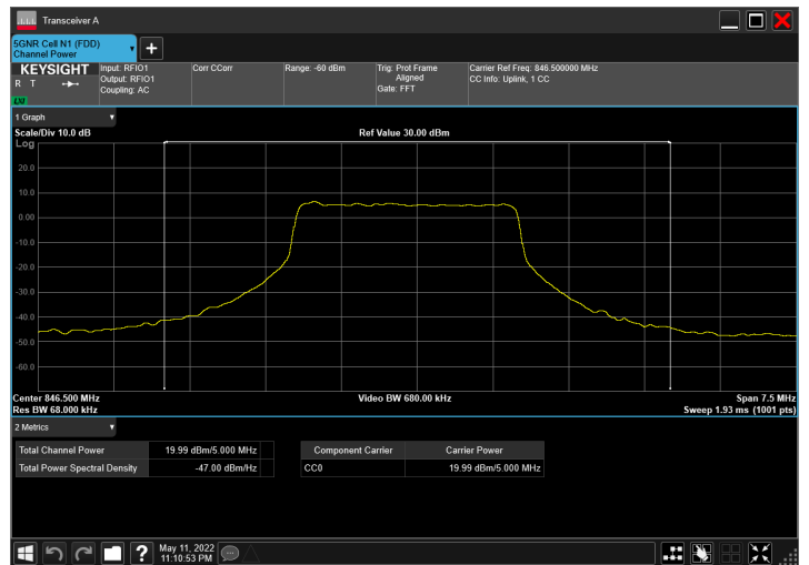
DC_2A_n5A_10MHz|5MHz_15kHz_1905MHz|846.5MHz_QPS K|CP-OFDM QPSK_RB12@0|RB13@6
