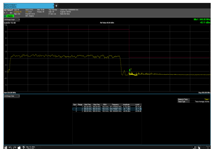
n5_15MHz_15kHz_841.5MHz_DFT-s-OFDM QPSK_RB75@0
