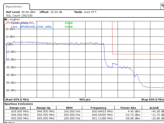
20MHz_15kHz_839MHz_DFT-s-OFDM QPSK_RB100@0 -24.72 dBm
