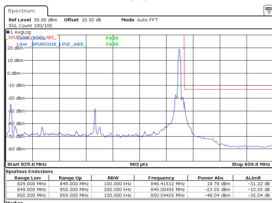
20MHz_15kHz_839MHz_DFT-s-OFDM QPSK_RB1@105 -23.05 dBm
