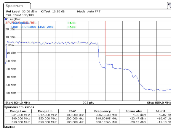
15MHz_15kHz_841.5MHz_DFT-s-OFDM QPSK_RB75@0 -23.47 dBm
