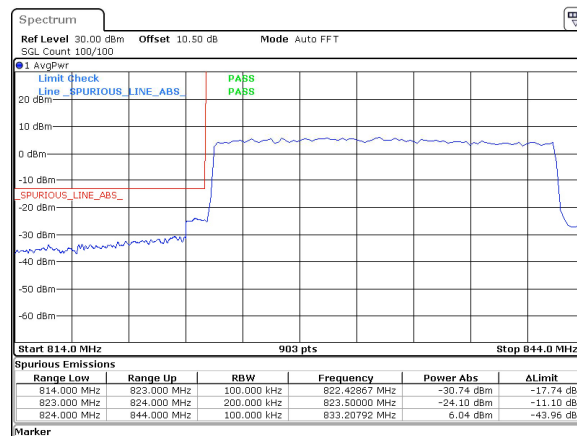
20MHz_15kHz_834MHz_DFT-s-OFDM QPSK_RB100@0 -24.10 dBm
