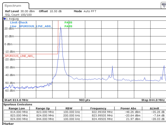
20MHz_15kHz_834MHz_DFT-s-OFDM QPSK_RB1@0 -20.64 dBm
