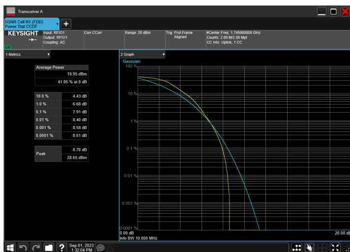
n66_10MHz_15kHz_1745MHz_DFT-s-OFDM QPSK_RB50@0
