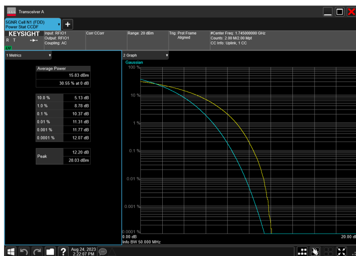
n66_40MHz_15kHz_1745MHz_CP-OFDM QPSK_RB216@0
