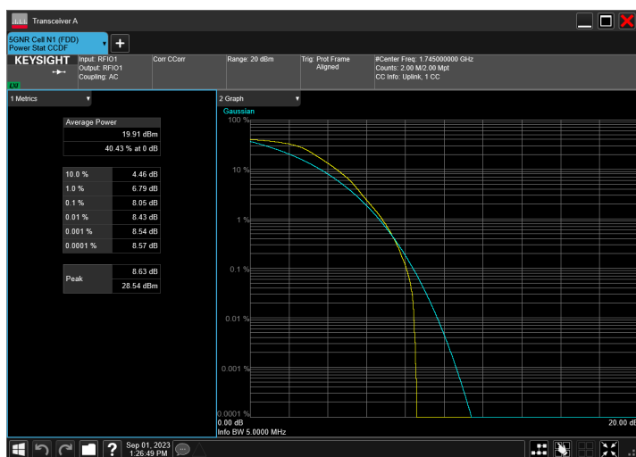
n66_5MHz_15kHz_1745MHz_DFT-s-OFDM QPSK_RB25@0
