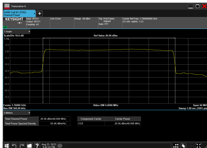
n66_40MHz_15kHz_1760MHz_DFT-s-OFDM QPSK_RB216@0
