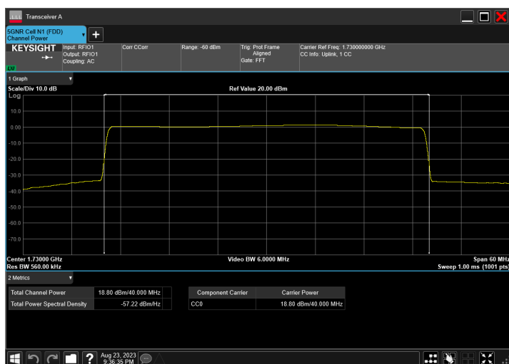
n66_40MHz_15kHz_1730MHz_CP-OFDM QPSK_RB216@0
