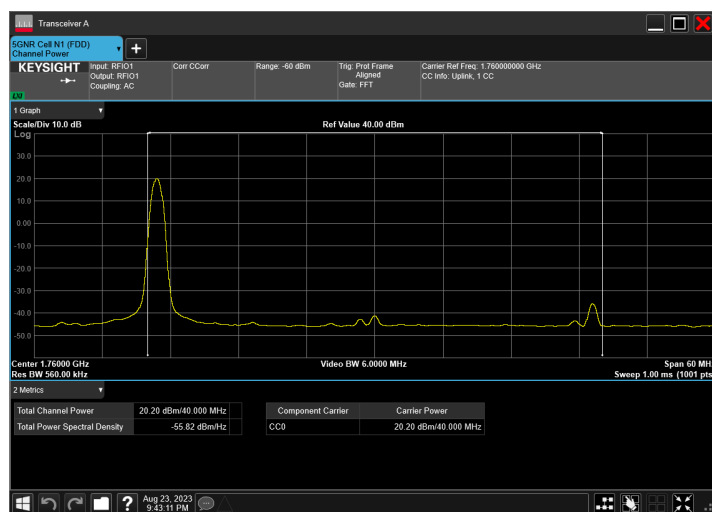
n66_40MHz_15kHz_1760MHz_CP-OFDM QPSK_RB1@1
