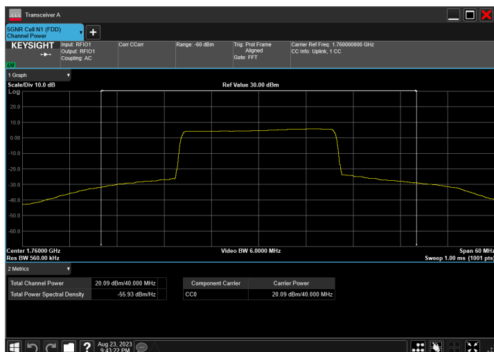
n66_40MHz_15kHz_1760MHz_CP-OFDM QPSK_RB216@0
