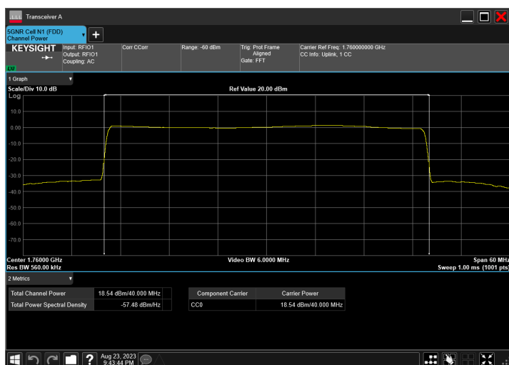
n66_40MHz_15kHz_1760MHz_CP-OFDM QPSK_RB216@0
