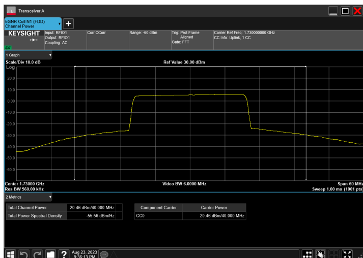
n66_40MHz_15kHz_1730MHz_CP-OFDM QPSK_RB216@0
