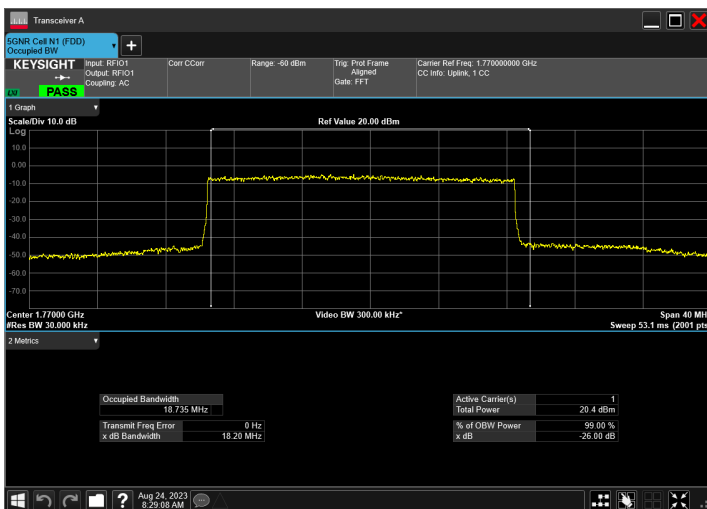
n66_20MHz_15kHz_1770MHz_DFT-s-OFDM QPSK_RB100@0
