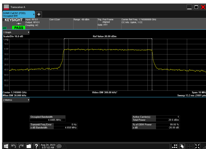
n66_5MHz_15kHz_1745MHz_DFT-s-OFDM QPSK_RB25@0
