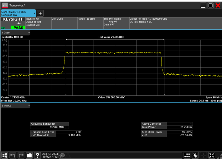
n66_10MHz_15kHz_1715MHz_DFT-s-OFDM QPSK_RB50@0
