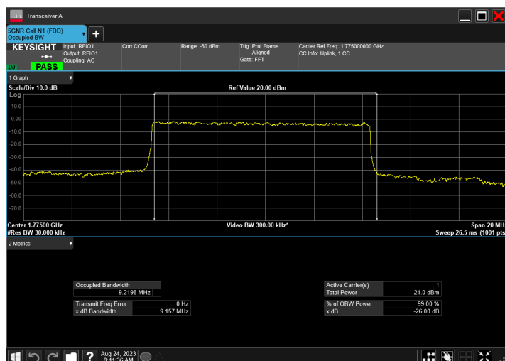
n66_10MHz_15kHz_1775MHz_DFT-s-OFDM PI/2 BPSK_RB50@0
