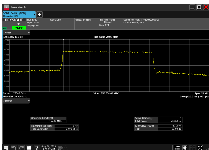
n66_10MHz_15kHz_1775MHz_DFT-s-OFDM QPSK_RB50@0
