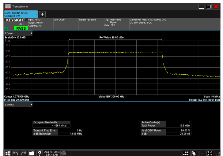
n66_5MHz_15kHz_1777.5MHz_CP-OFDM QPSK_RB25@0
