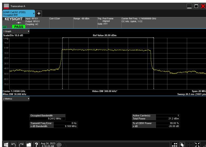
n66_10MHz_15kHz_1745MHz_DFT-s-OFDM PI/2 BPSK_RB50@0
