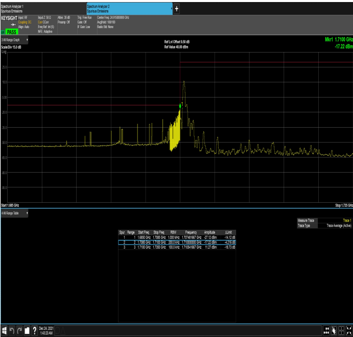
n66_20MHz_15kHz_1720MHz_DFT-s-OFDM QPSK_RB1@0
