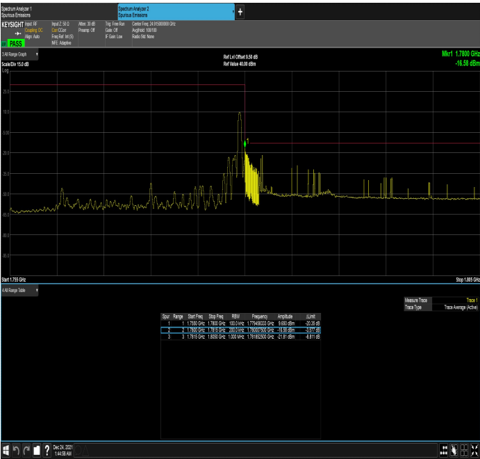
n66_20MHz_15kHz_1770MHz_DFT-s-OFDM QPSK_RB1@105
