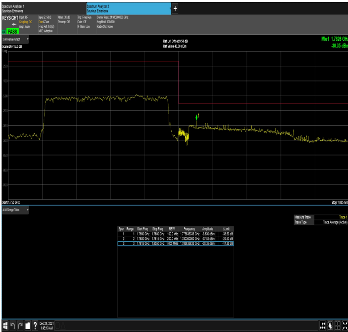
n66_20MHz_15kHz_1770MHz_DFT-s-OFDM QPSK_RB100@0
