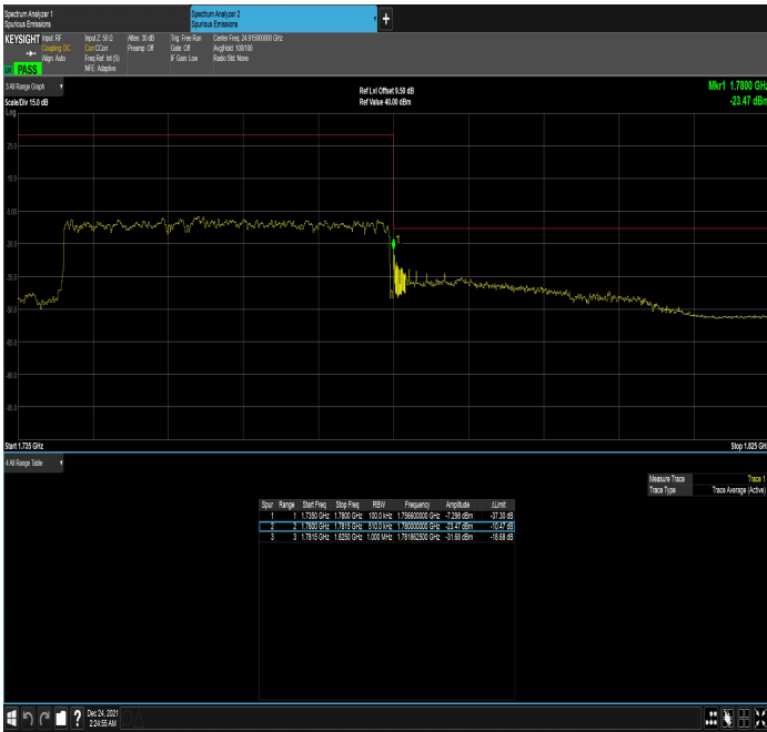
n66_40MHz_15kHz_1760MHz_DFT-s-OFDM QPSK_RB216@0
