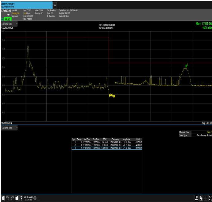
n66_20MHz_15kHz_1770MHz_DFT-s-OFDM QPSK_RB1@0
