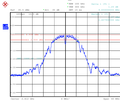
802.11b_2412MHz
