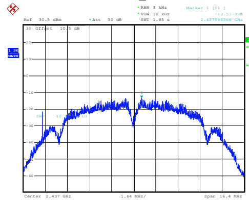
802.11b_2437MHz
