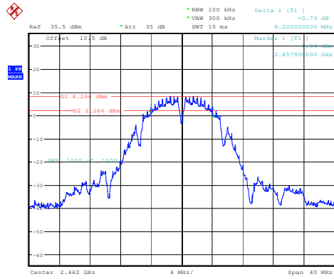
802.11b_2462MHz
