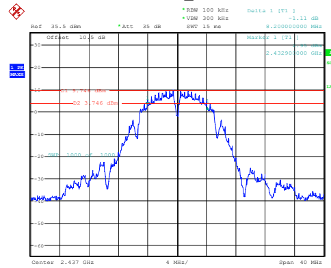
802.11b_2437MHz
