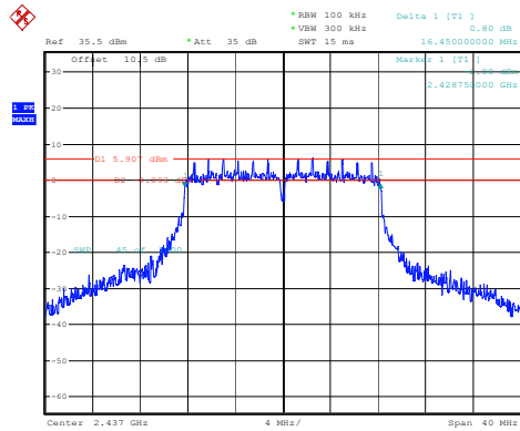
802.11g_2437MHz
