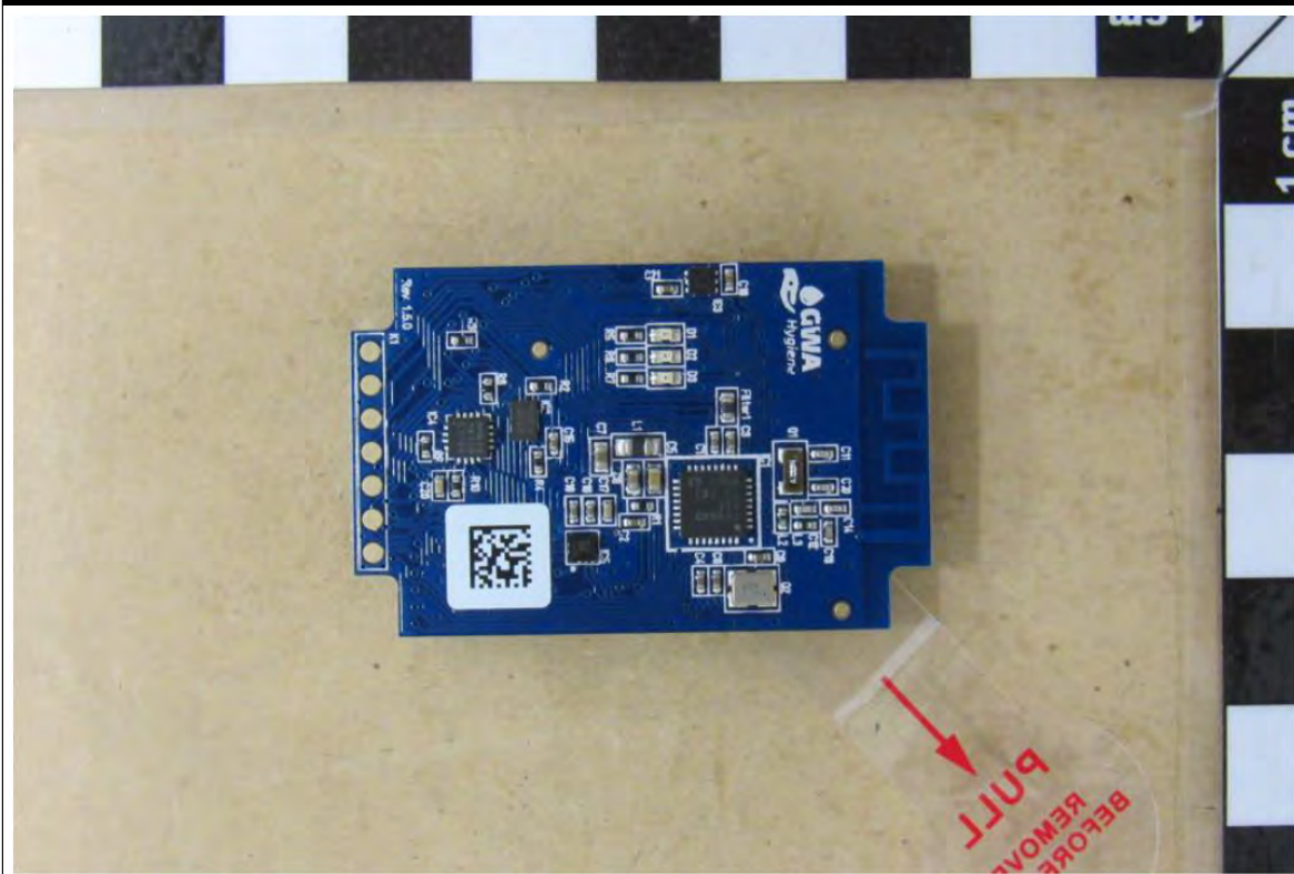
Sensormodul PCB bottom
