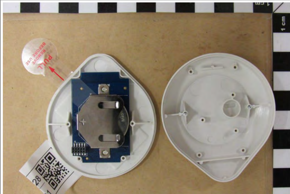
SensorModul PCB top
