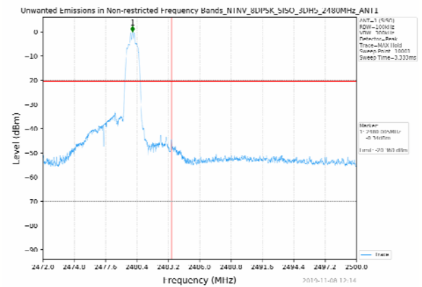
Right Band edge hopping off
