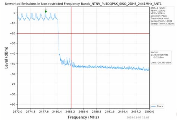
Right Band edge hopping on
