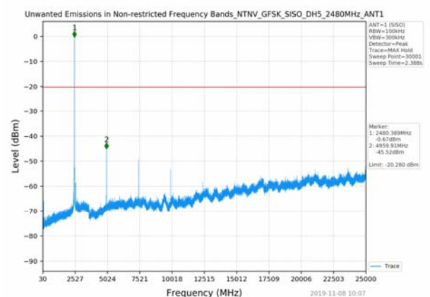
CH78 30MHz-25GHz
