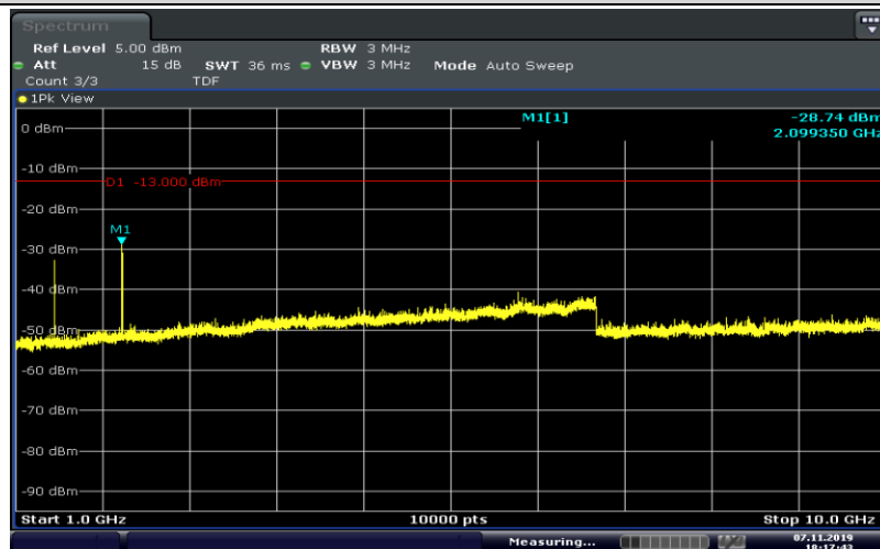
Band12-1.4MHz-QPSK-23017-6RB#0-Range2:1000~10000MHz
