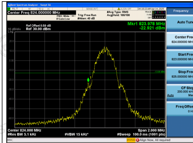
GSM850-128-5-PASS
