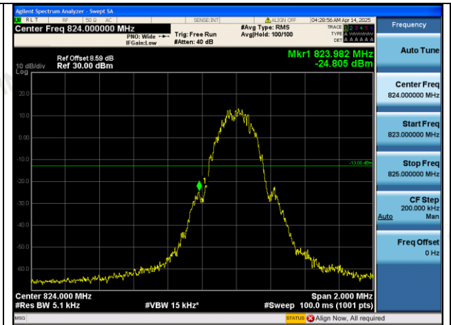
GPRS850-128-5-PASS
