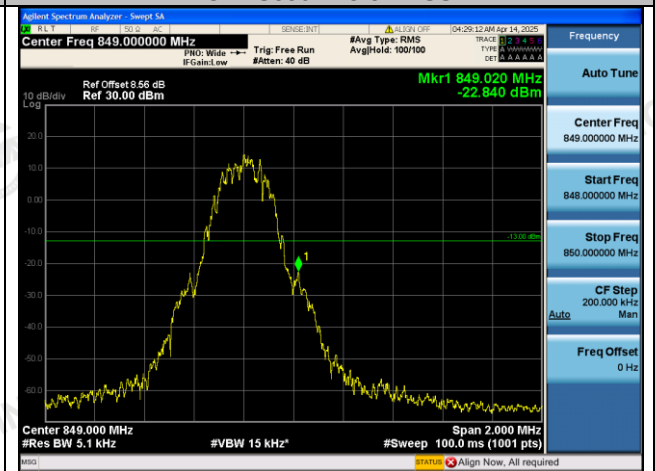
GPRS850-251-5-PASS
