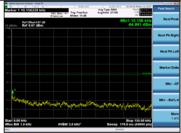
20MHz_MCH_QPSK_1RB#0
