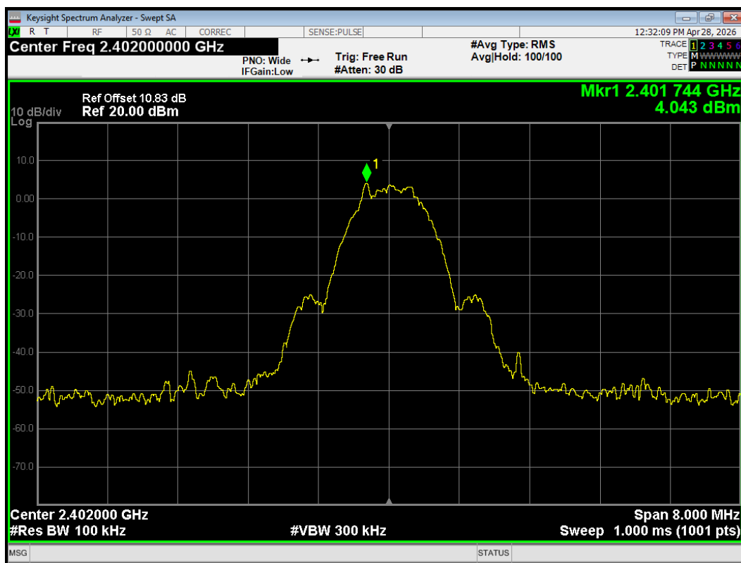
Band Edge BLE 2402MHz Emission
