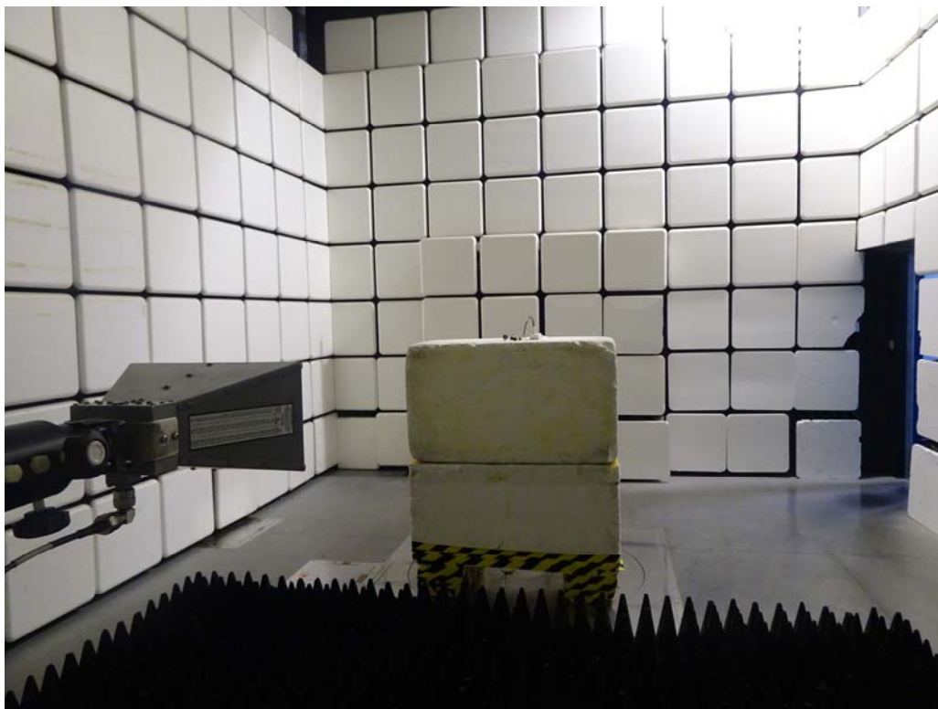
1GHz-18GHz
