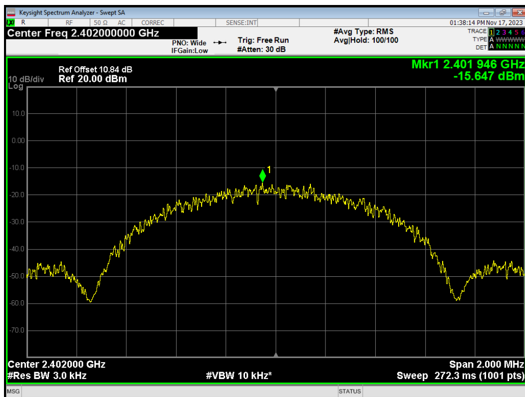
PSD Bluetooth LE 2402MHz
