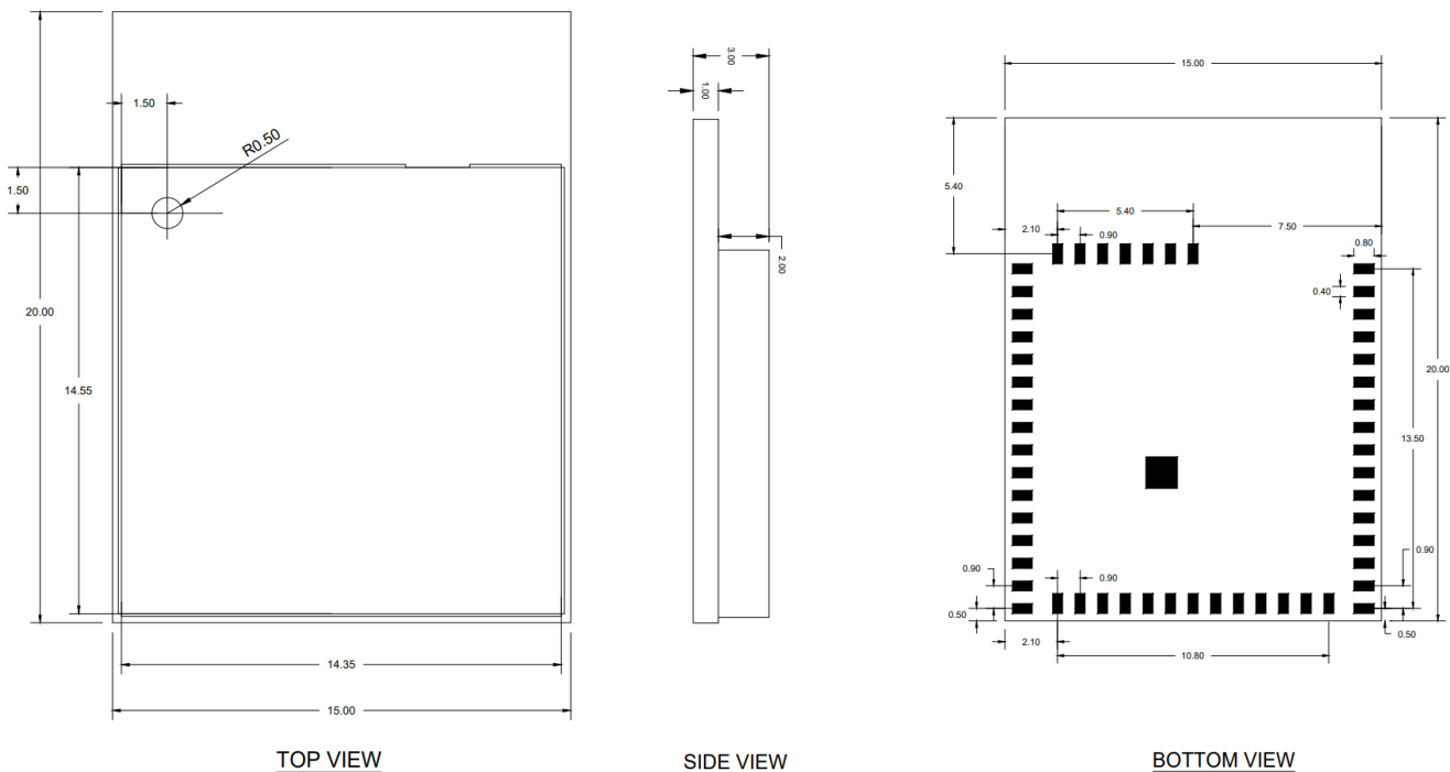
Figure 26. RRQ61051-008 module dimensions
