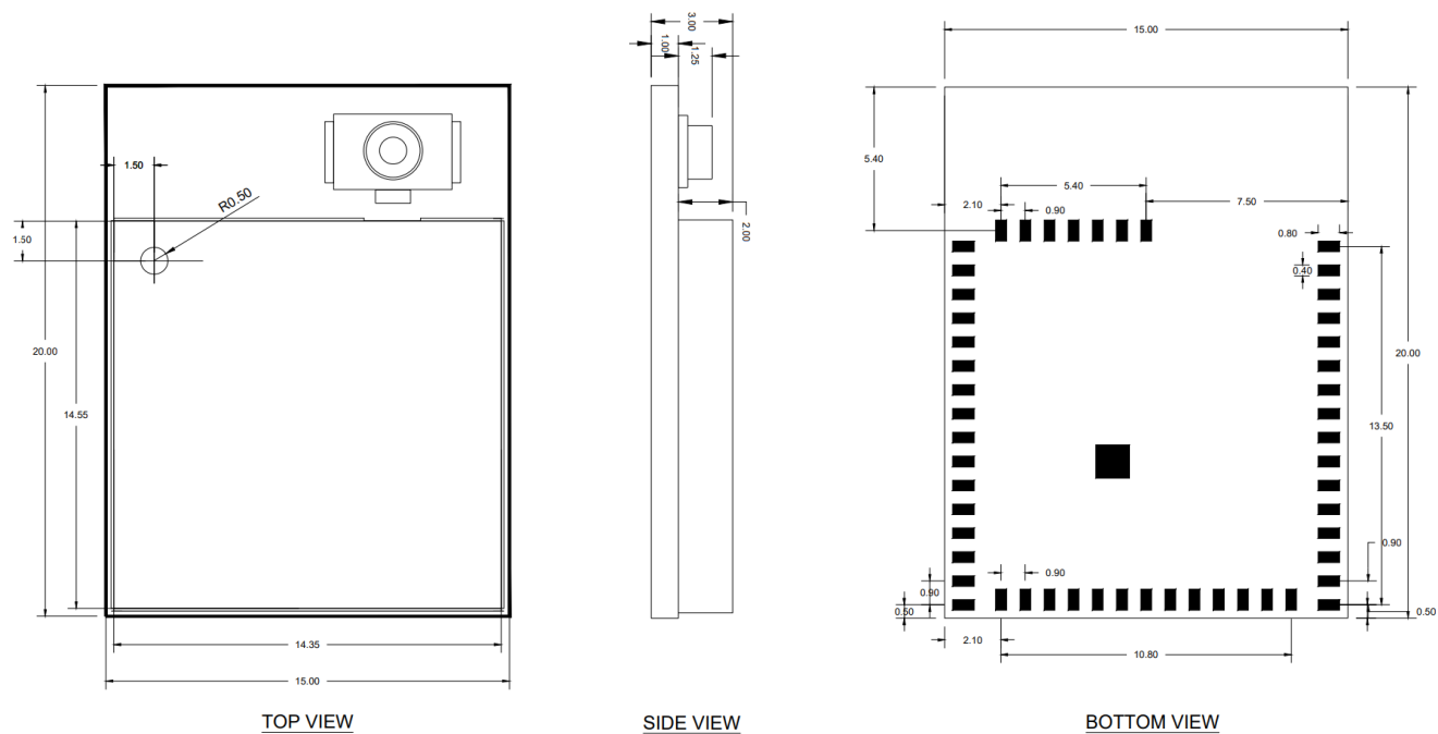
Figure 25. RRQ61051-009 module dimensions
