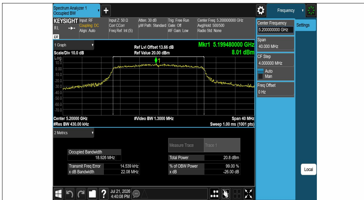
11AX20SISO-Ant1-5200
