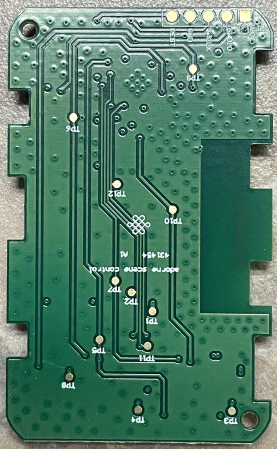
PCBA - BOT
