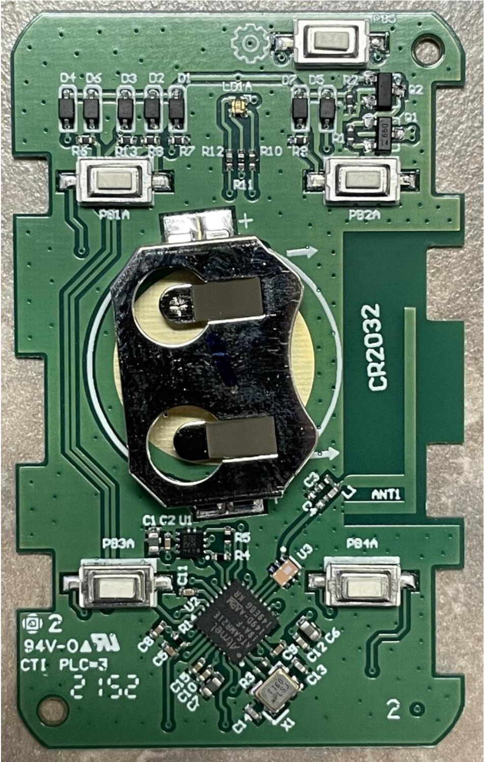
PCBA - TOP
