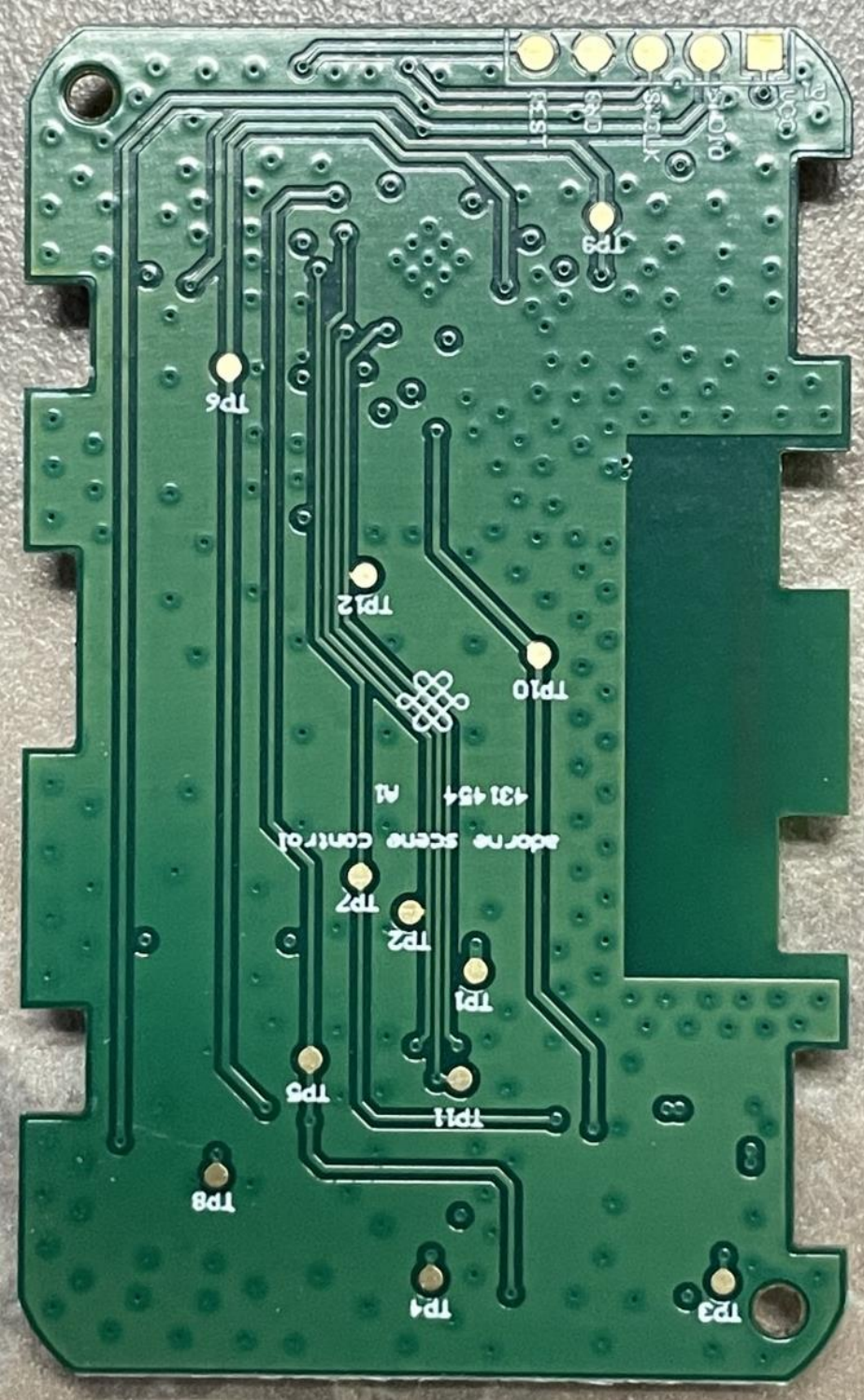
PCBA - BOT
