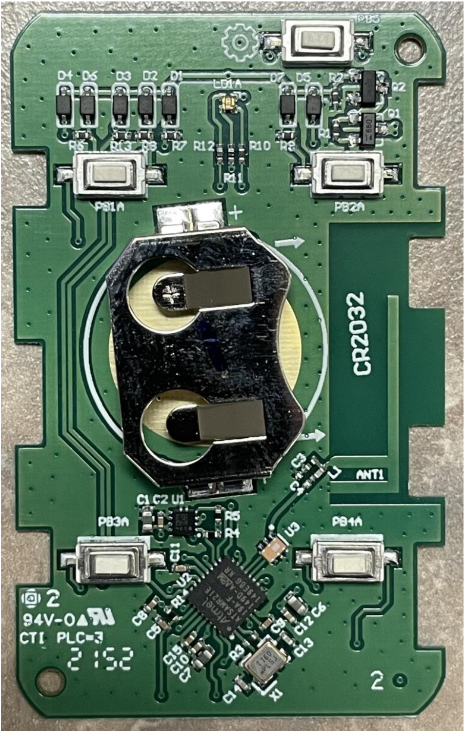
PCBA - TOP
