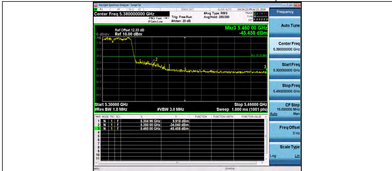
11AC40MIMO_Ant1_Low_5510_AV
