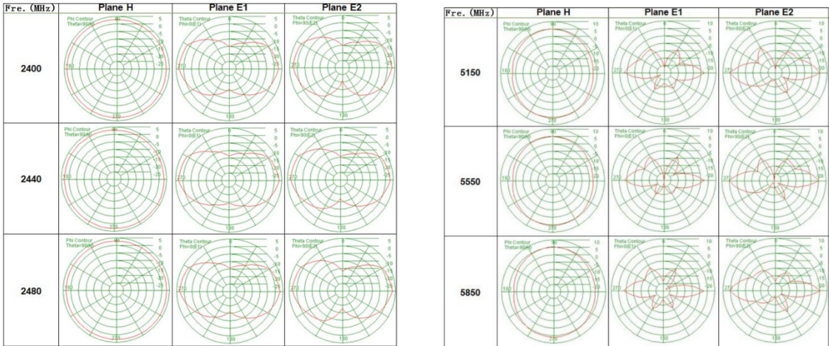
双频天线极化方向图
