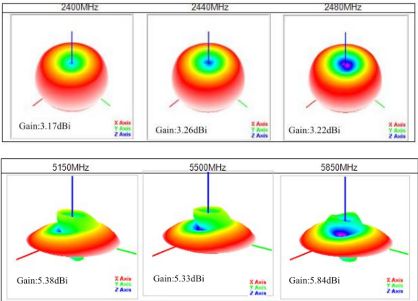
双频天线辐射方向图
