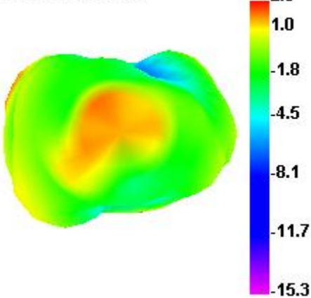
2500.000MHz
