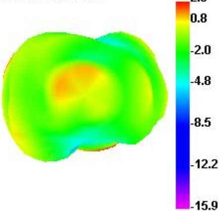
2450.000MHz
